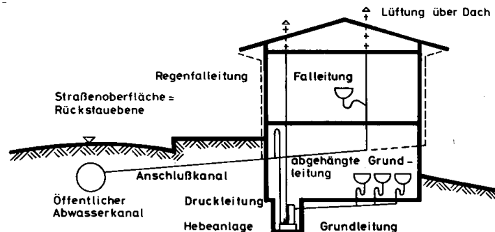
Schema für eine Hebeanlage in der Grundstücksentwässerung
